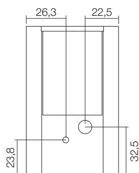
vista retro stufa
